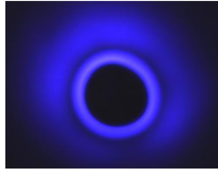
Image d'un plasmöide
