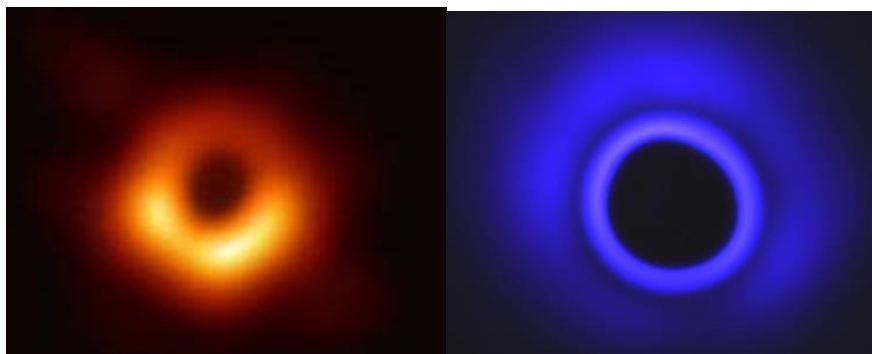
Изображение «черной дыры». Изображение «плазмоида».
