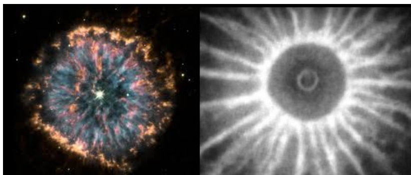
Светящаяся небула глаза NGC 6751. Показывается, как из центральной звезды выбрасывается плазма.
